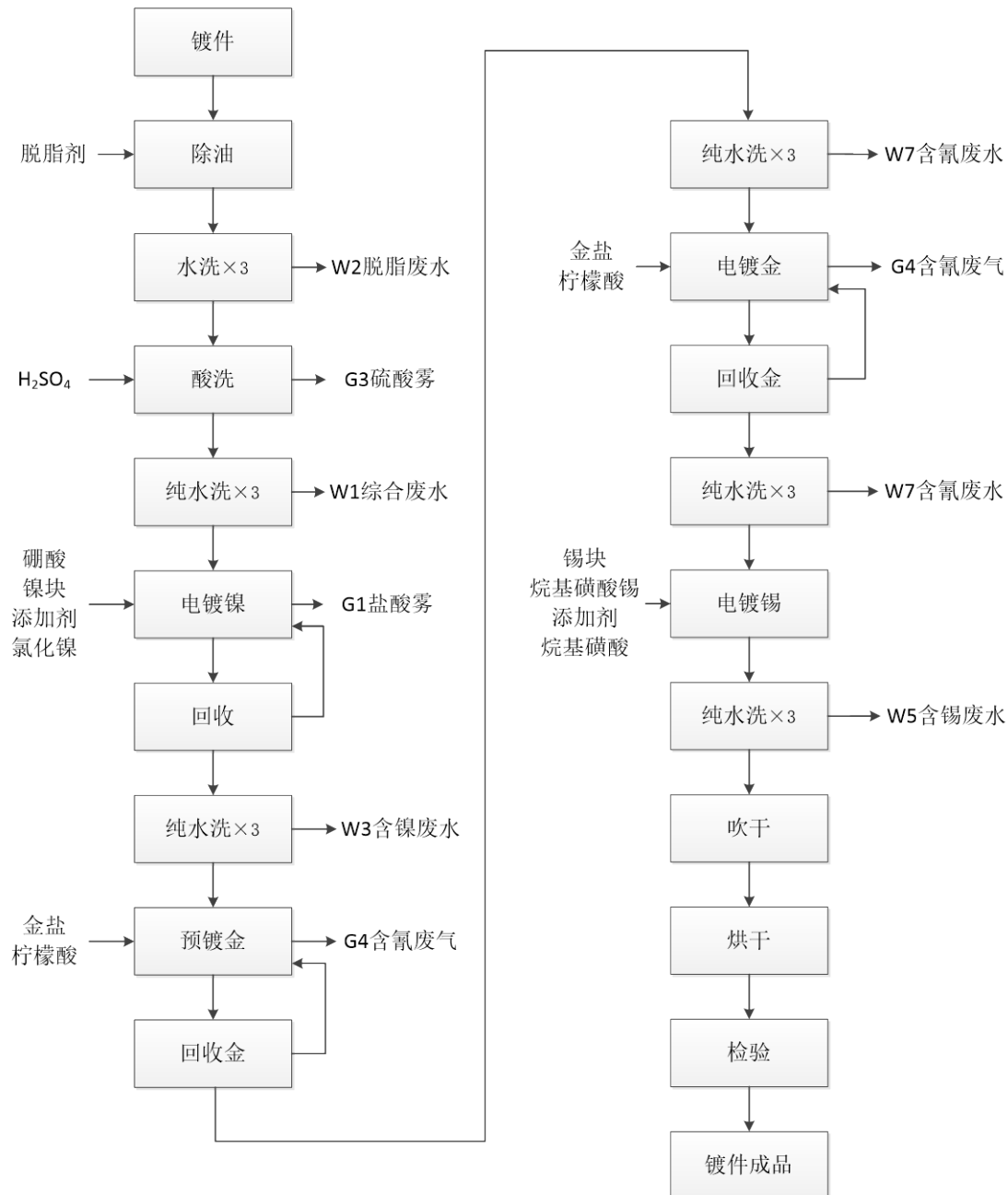
图 2.4-2 端子电镀镍、金、锡工艺产污环节
