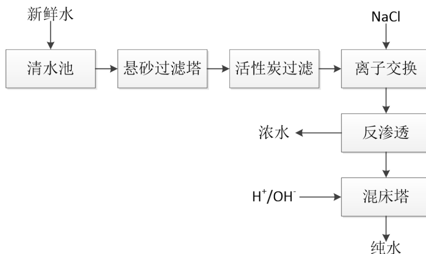
图 2.3-2 纯水制备工艺流程
