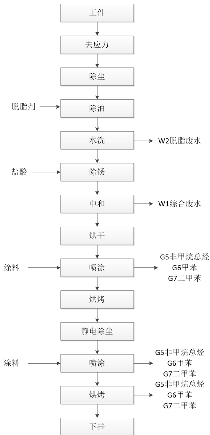
图 2.4-10 低温烤漆工艺产污环节
