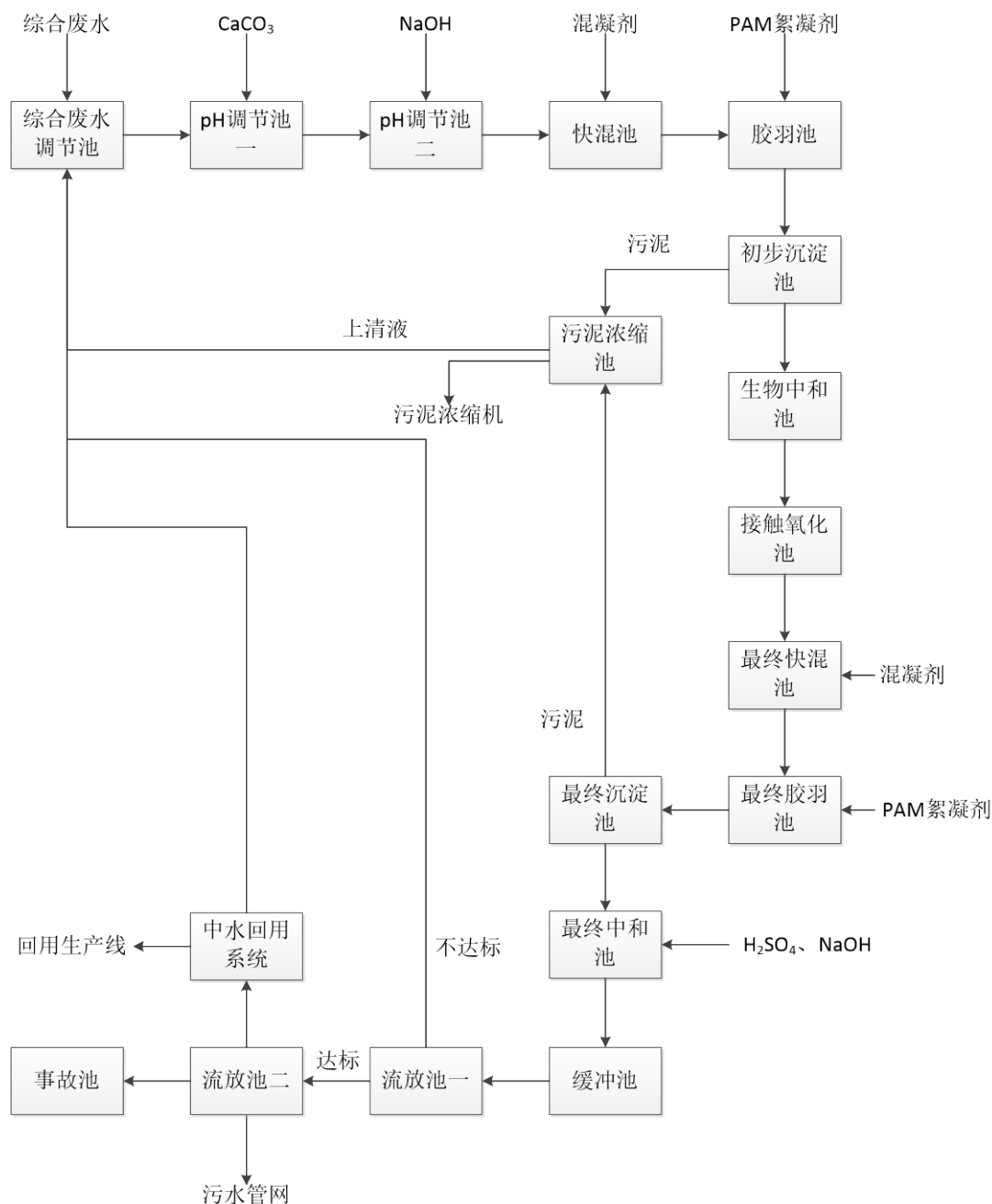
图 5.3-7 综合废水处理系统流程图
