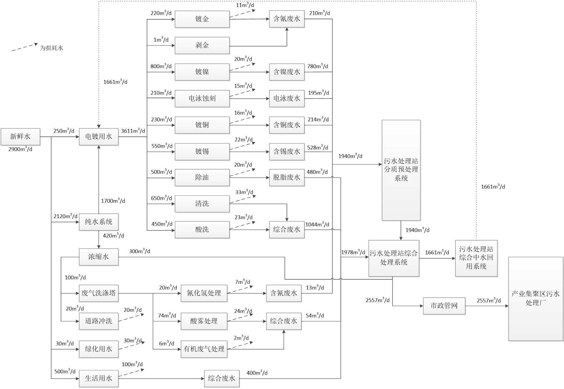
图 2.3-1 项目用水平衡图
