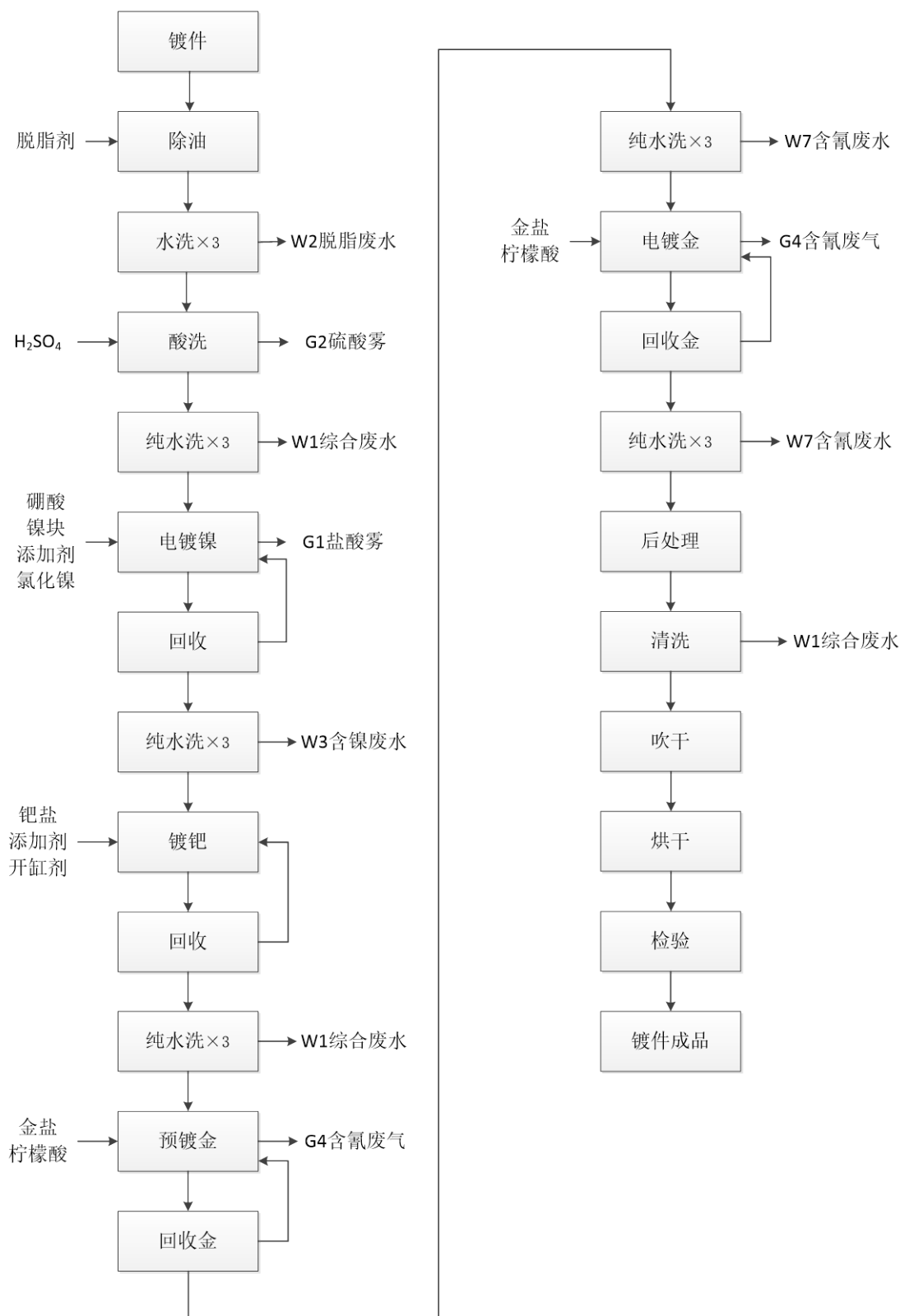
图 2.4-3 端子线电镀镍、钯、金工艺产污环节
