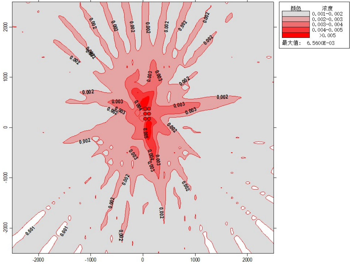
图 4.1-5 评价区域盐酸雾小时浓度最大值分布图
