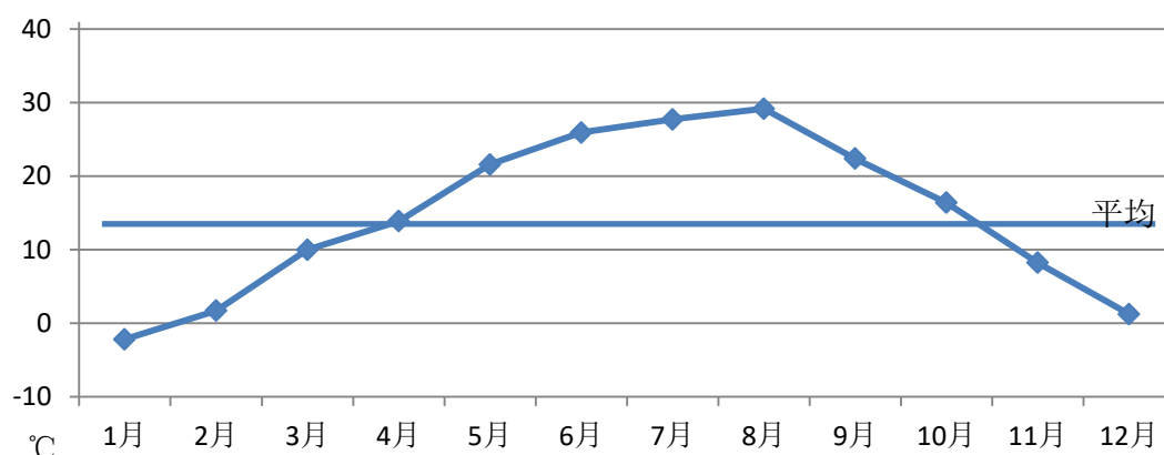
图 4.1-1 平均气温月变化曲线
