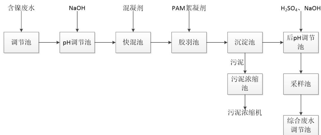
图 5.3-2 含镍废水预处理单元流程图
