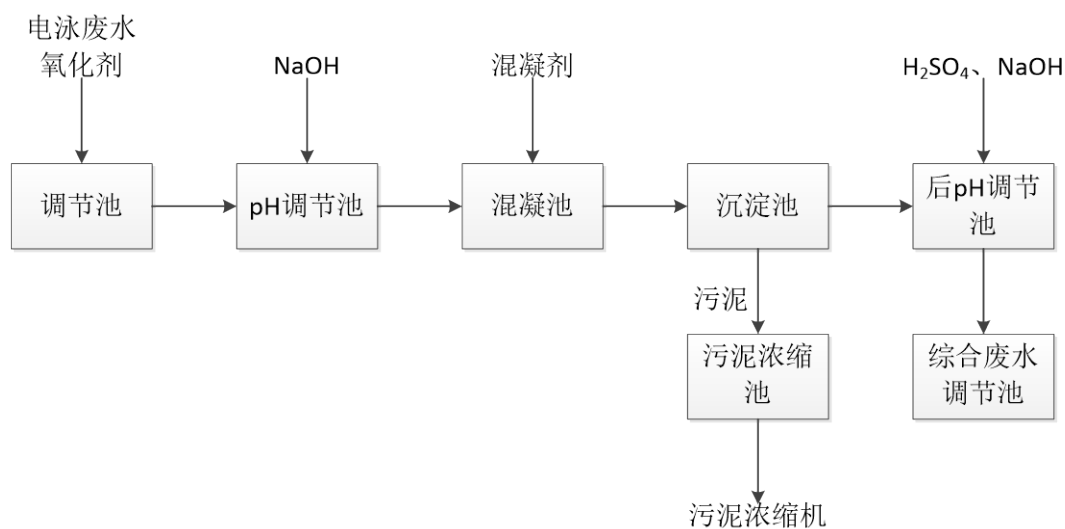
图 5.3-6 电泳废水预处理单元流程图
