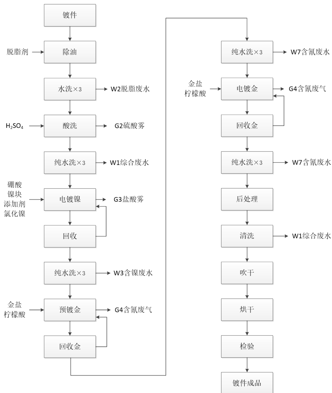
图 2.4-4 端子线电镀镍、金工艺产污环节
