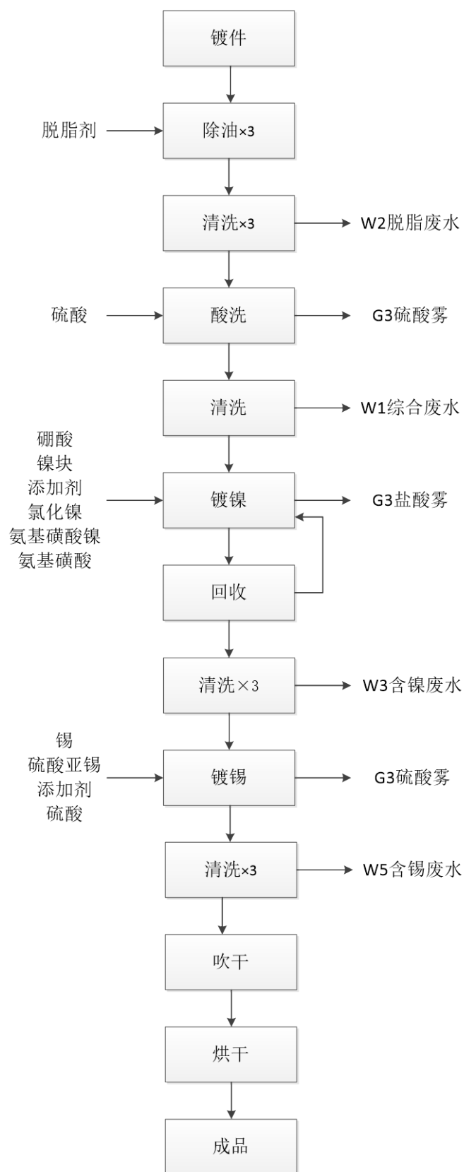
图 2.4-5 滚镀镀镍工艺产污环节
