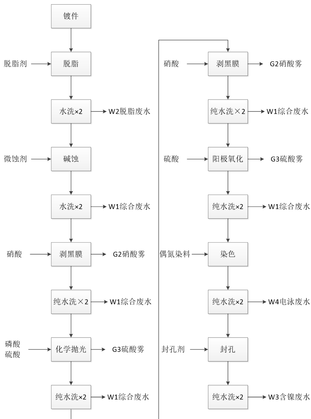
图 2.4-9 阳极氧化工艺产污环节
