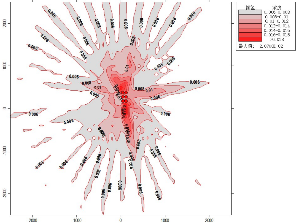
图 4.1-4 评价区域硫酸雾小时浓度最大值分布图
